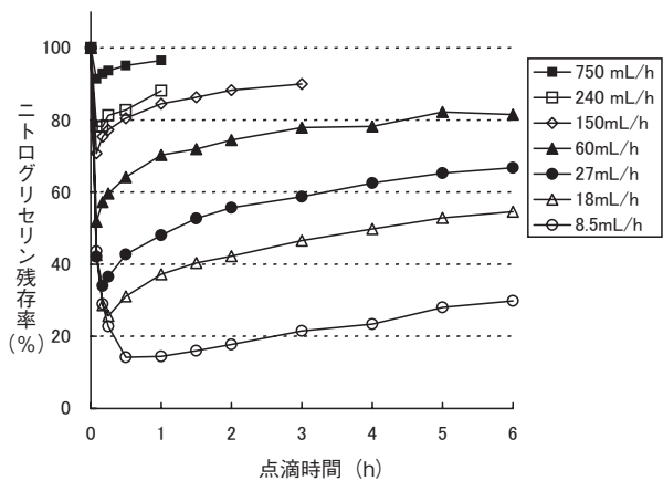
点滴速度によるニトログリセリン残存率への影響 測定条件：室温 塩化ビニル管の長さ：120cm
